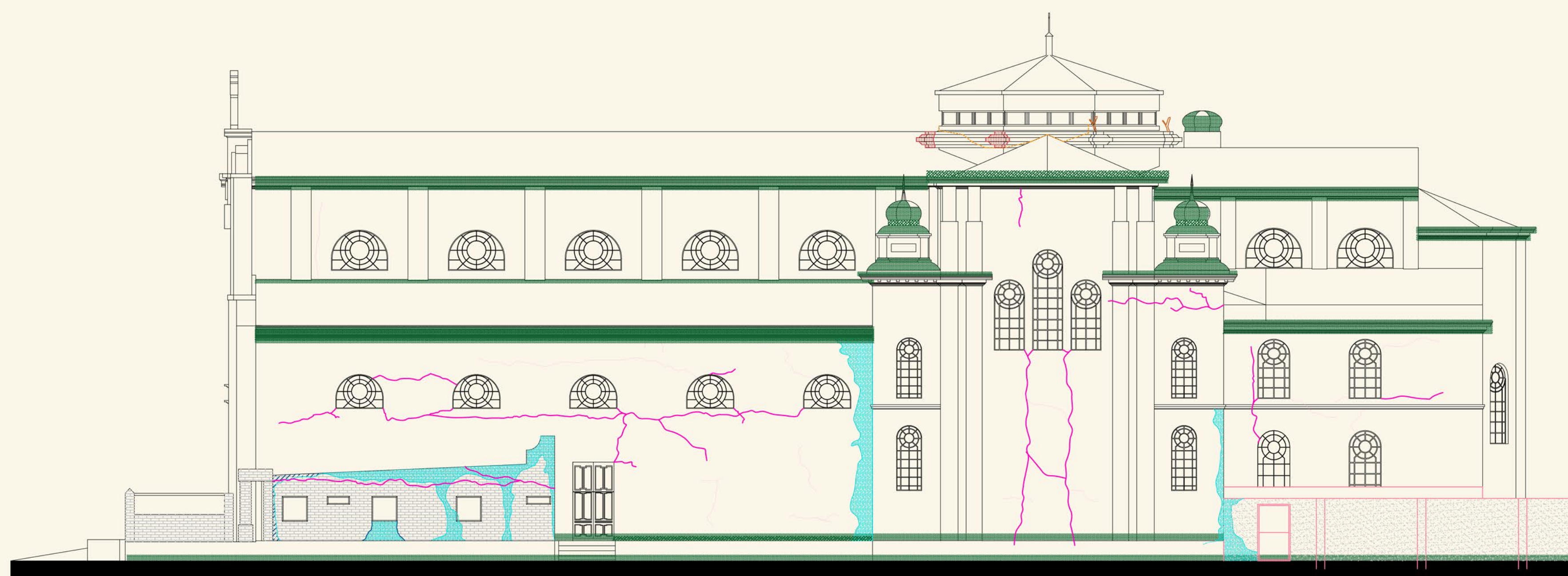
ELEVACIÓN LONGITUDINAL PONIENTE
