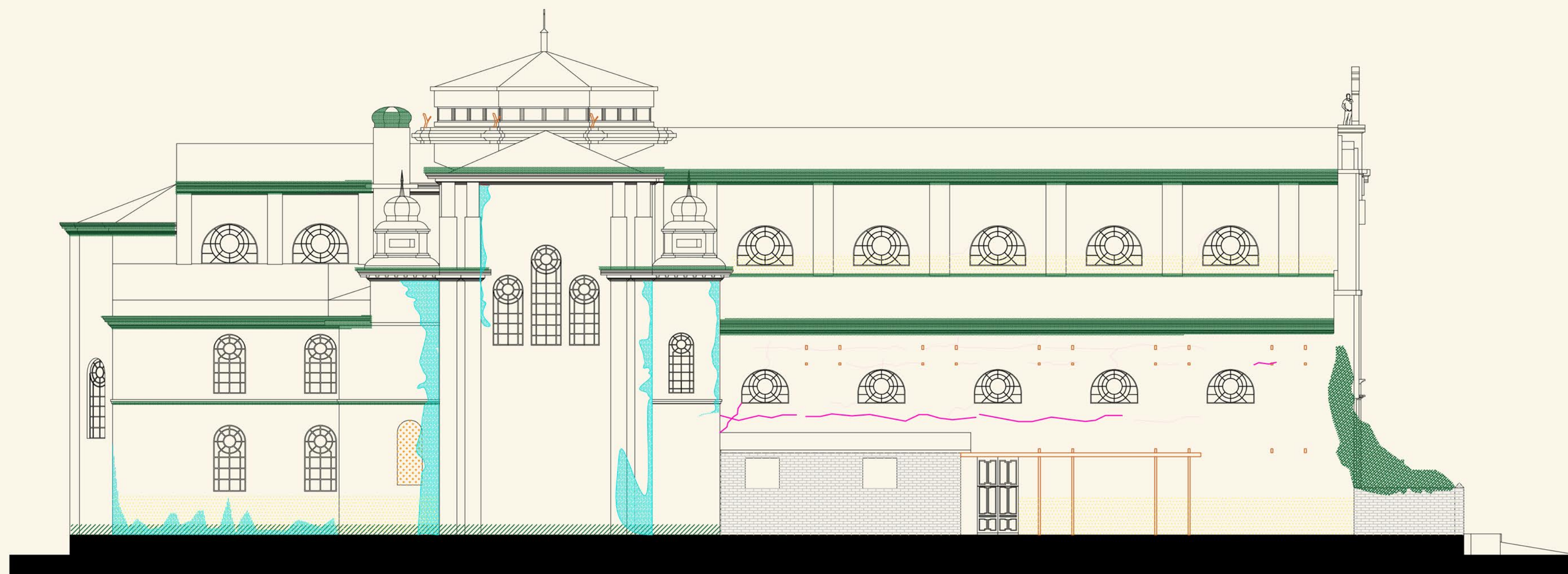
ELEVACIÓN LONGITUDINAL ORIENTE
