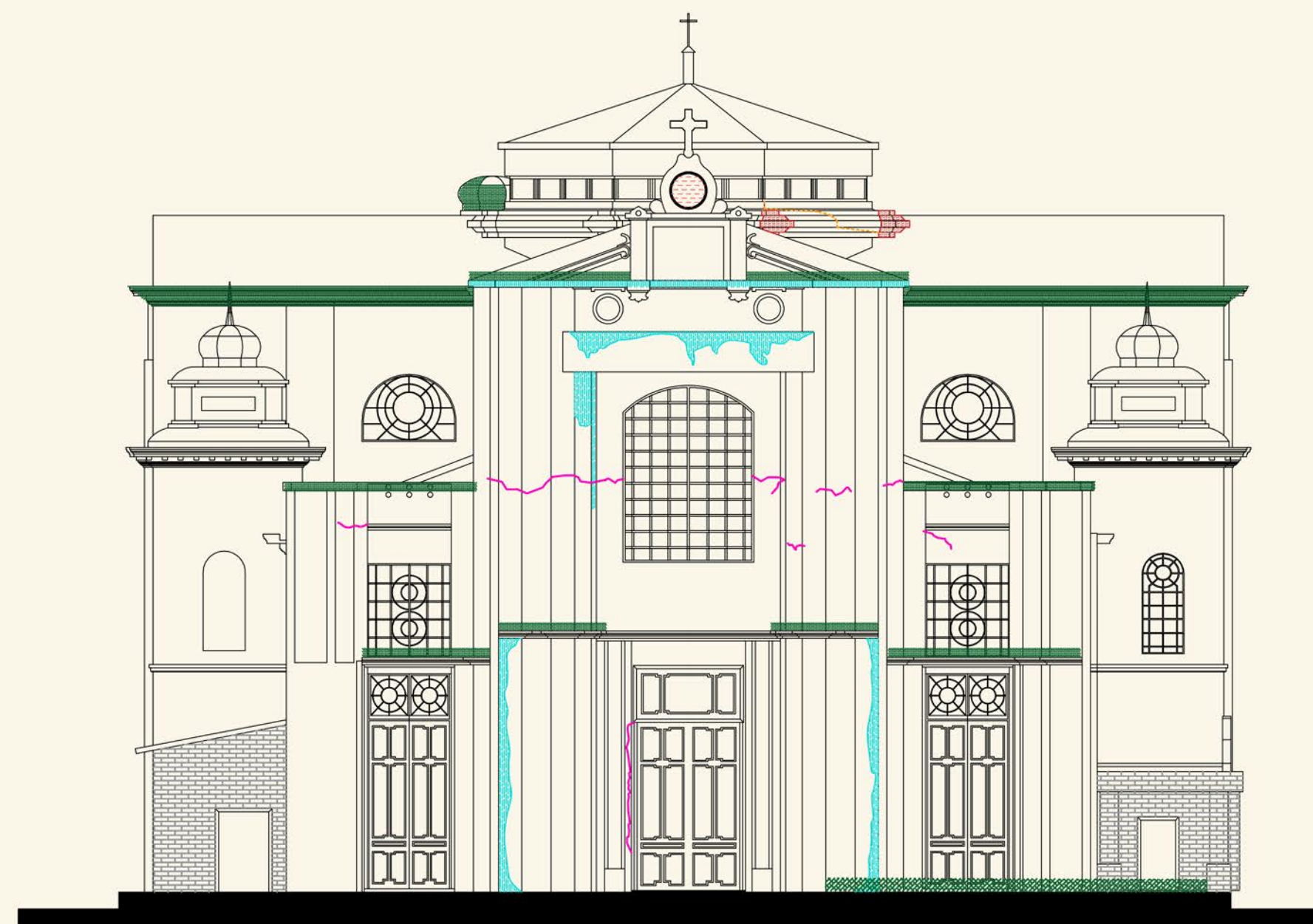
ELEVACIÓN FRONTAL
